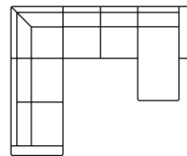
U corner (R) Art.No.:14400 H88 x D242 x W349cm
